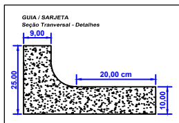
PAVIMENTAÇÃO: Seção Transversal - Detalhes
