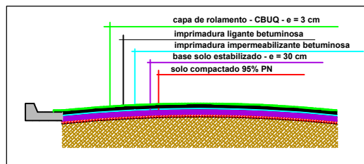
PAVIMENTAÇÃO: Seção Transversal - Detalhes
